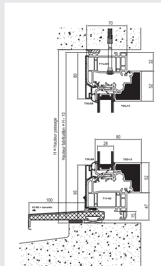
Pièce d'appui de 100 mm en base
