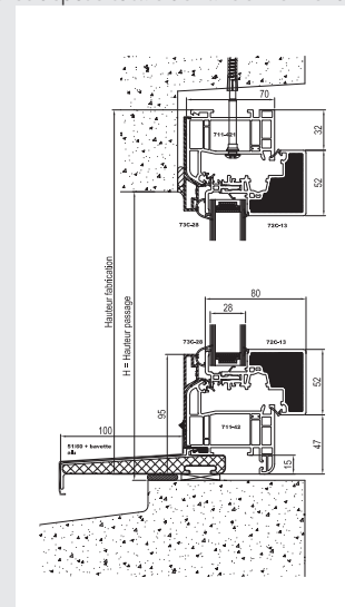
Dormant de 70 mm et pièce d'appui rapportée dépassant de 100 mm
